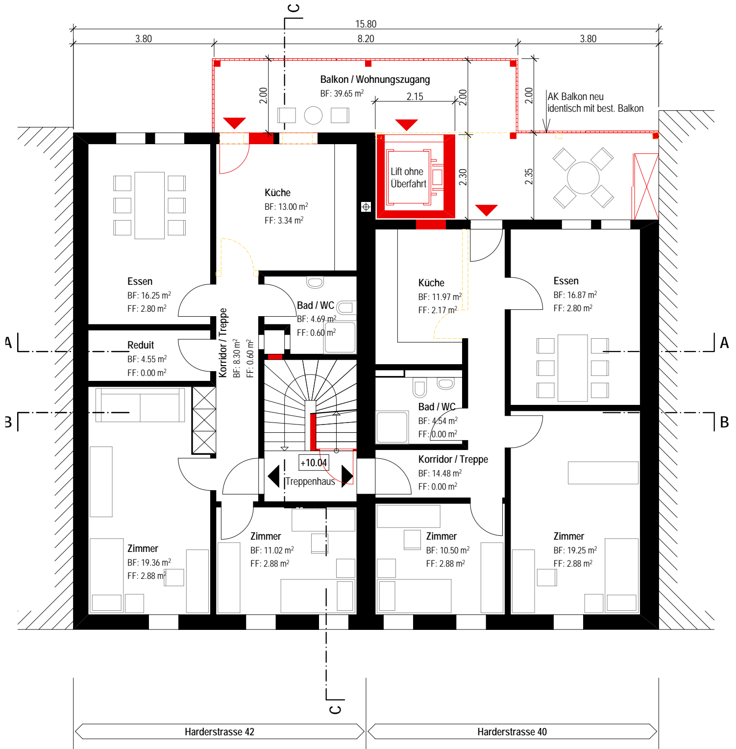
Grundriss 3. OG
